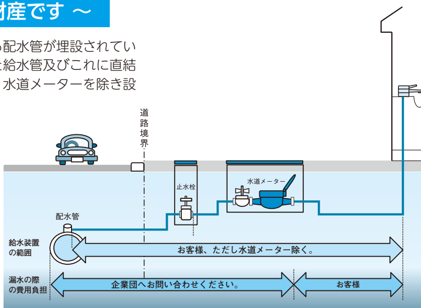
▲給水装置の概略図（家庭の場合）
