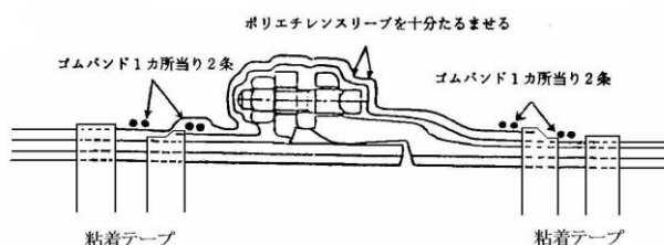
図 1-2 継手部の施工方法
