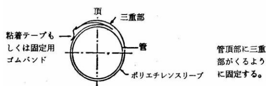
図 1-1 スリーブ固定法
